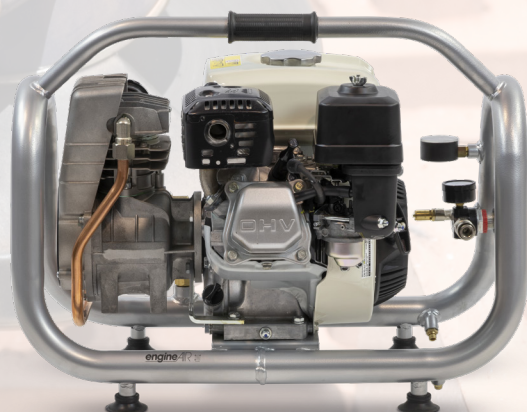
engineAIR 5/2,5 10 BENZIN
